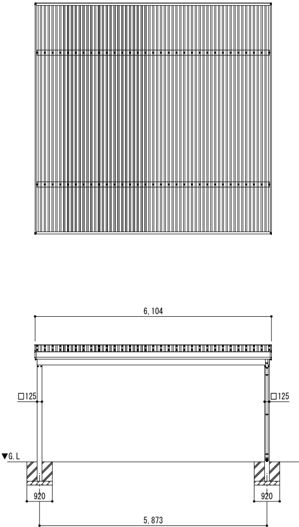
■姿図
