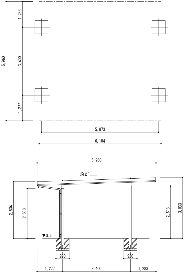
■基礎配置図
